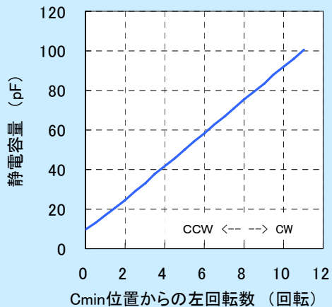
回転数—静電容量 特性
