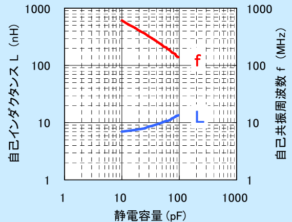
静電容量—自己インダクタンス・周波数 特性
