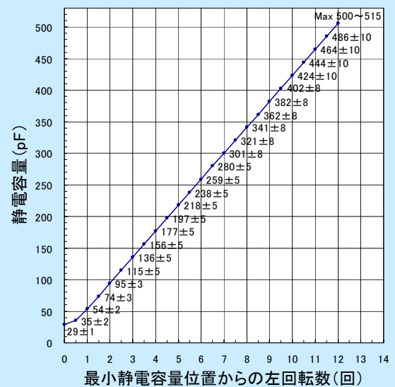
回転数-静電容量 特性
