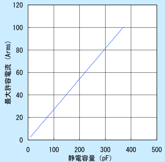
静電容量-電流 特性
