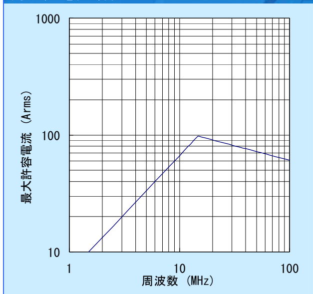
周波数-電流 特性
