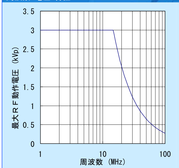
周波数-電圧 特性
